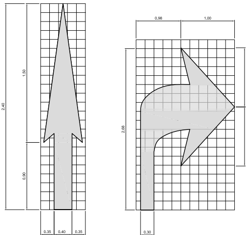
DETALLE "3" FLECHAS REFLECTANTES COLOR BLANCO S/ ESC.
